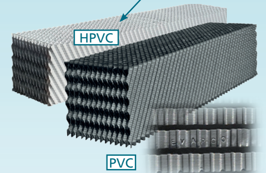
Counterflow Deck Fill Pacco di Scambio Surface d'Echange à Courants Croisés Fullkörper
